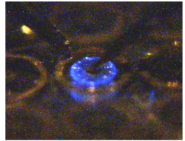
図1. 世界で初めて光ったZnO紫外発光ダイオード(LED)
